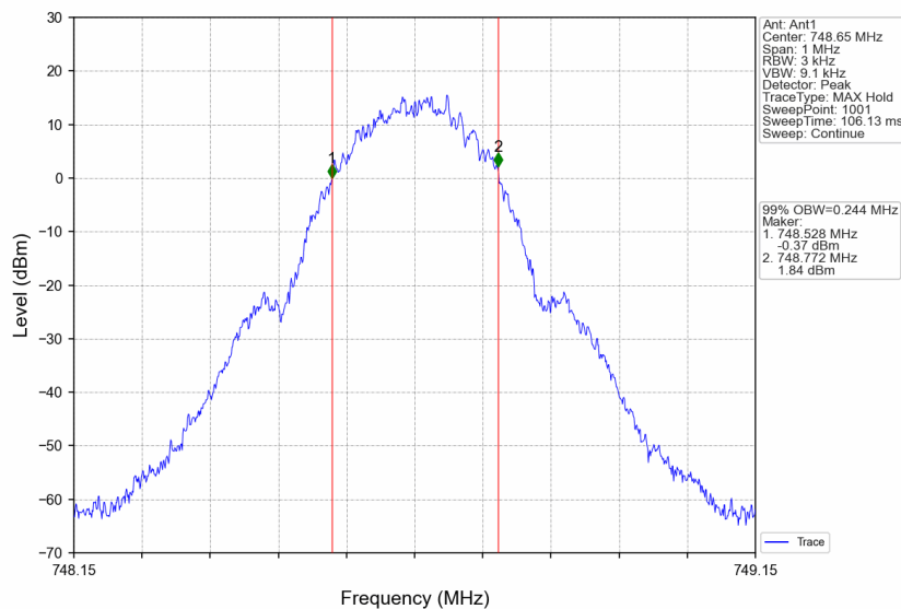
Band13_748.65MHz_GMSK_SISO_Ant1_NTNV_AGC
