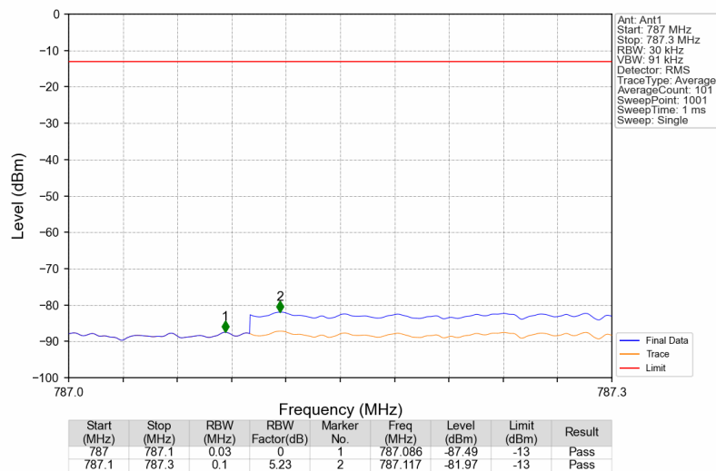
Band13_755.9MHz_GMSK_SISO_Ant1_NTNV_AGC+3
