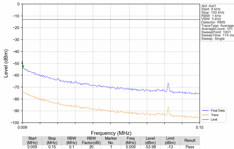
Band13_751MHz_AWGN_SISO_Ant1_NTNV
