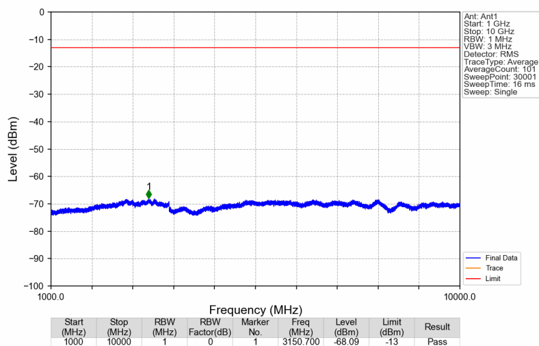
Band13_755.9MHz_GMSK_SISO_Ant1_NTNV
