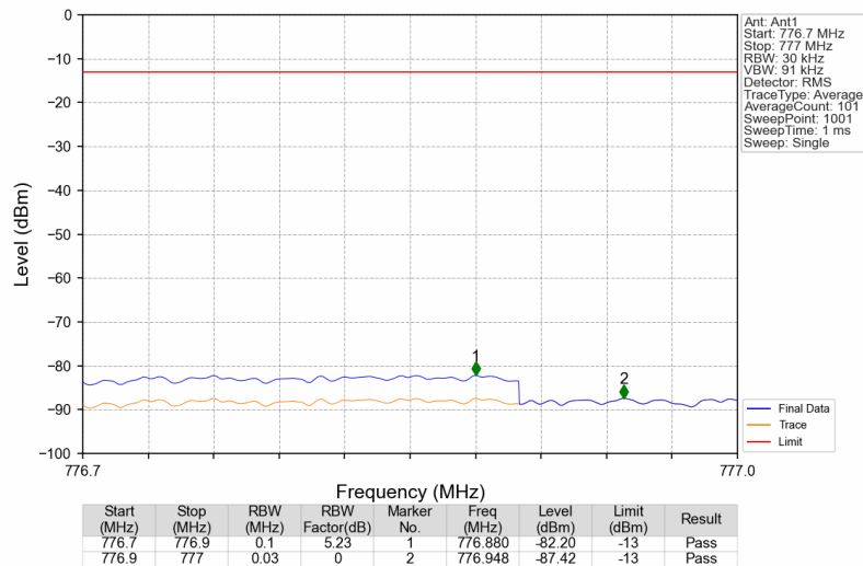
Band13_746.1MHz_GMSK_SISO_Ant1_NTNV_AGC+3
