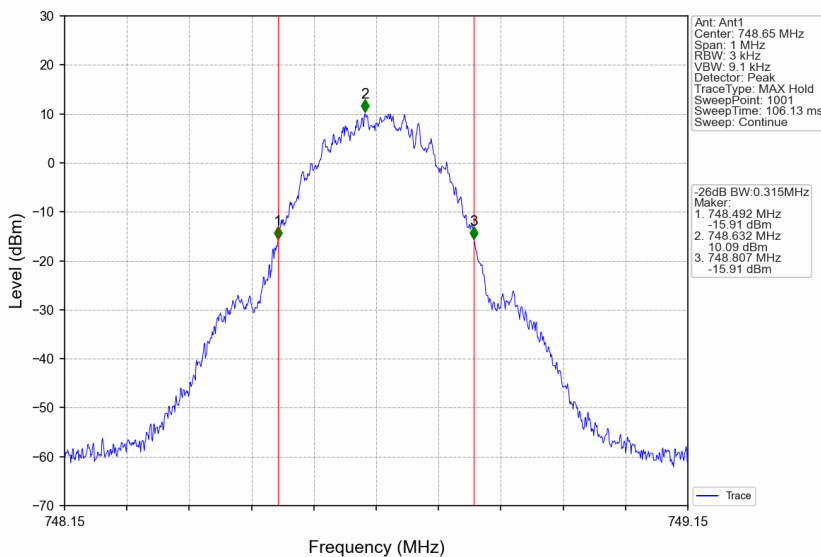
Band13_748.65MHz_GMSK_SISO_Ant1_NTNV_AGC+3
