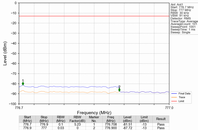
Band13_746.1MHz_GMSK_SISO_Ant1_NTNV_AGC
