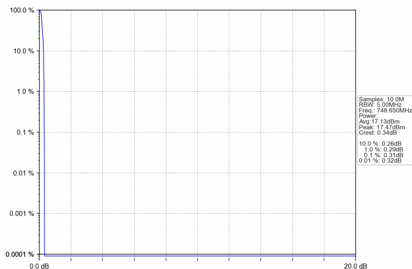
Band13_748.65MHz_GMSK_SISO_Ant1_NTNV_AGC+3
