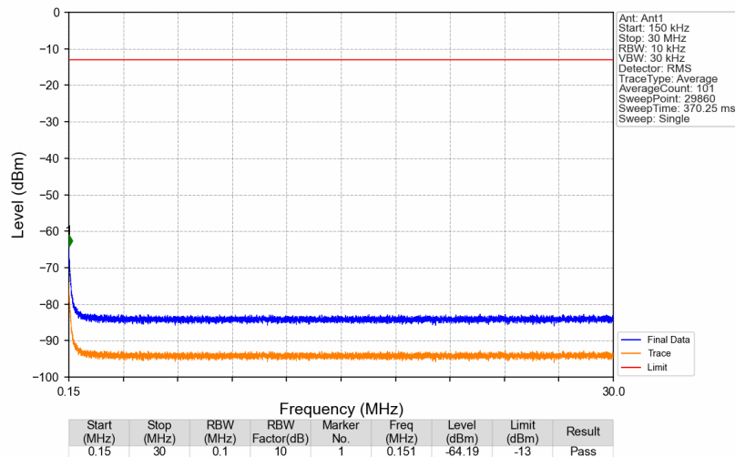
Band13_751MHz_GMSK_SISO_Ant1_NTNV
