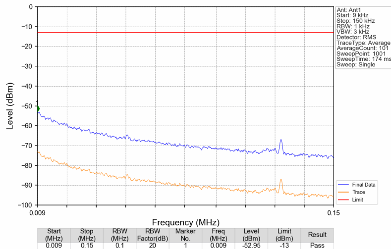
Band13_755.9MHz_GMSK_SISO_Ant1_NTNV
