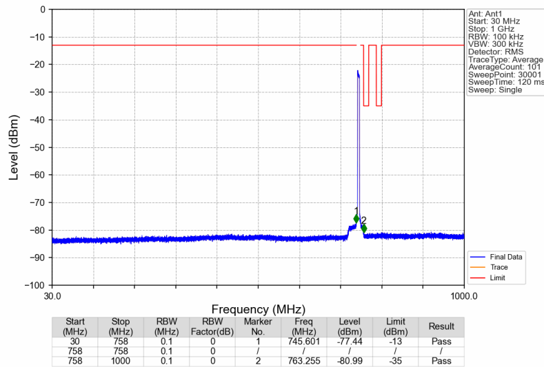
Band13_751MHz_AWGN_SISO_Ant1_NTNV
