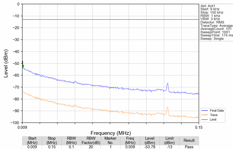
Band13_746.1MHz_GMSK_SISO_Ant1_NTNV
