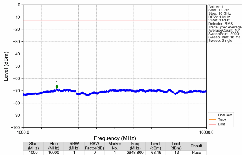
Band13_751MHz_AWGN_SISO_Ant1_NTNV
