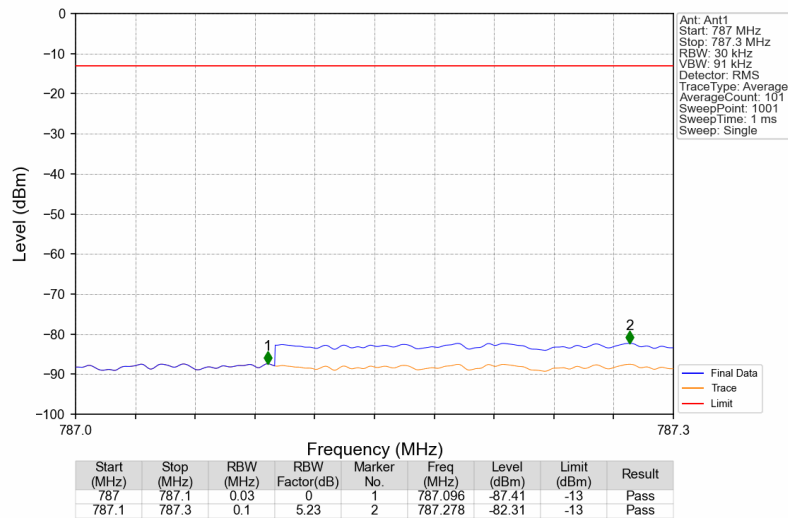
Band13_755.9MHz_GMSK_SISO_Ant1_NTNV_AGC
