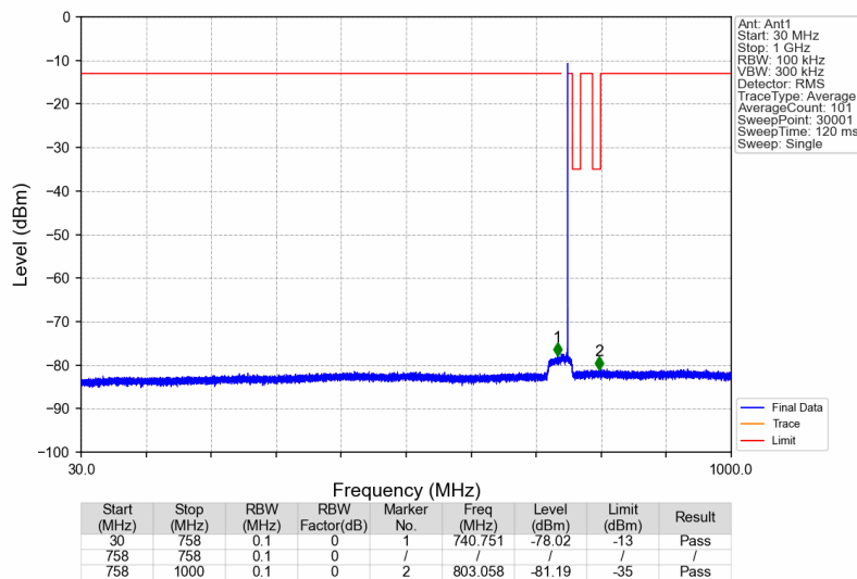
Band13_755.9MHz_GMSK_SISO_Ant1_NTNV
