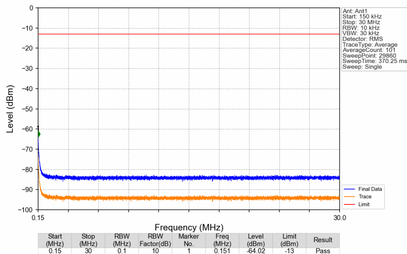
Band13_751MHz_AWGN_SISO_Ant1_NTNV
