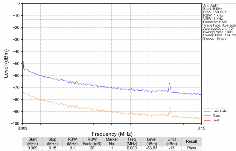
Band13_751MHz_GMSK_SISO_Ant1_NTNV
