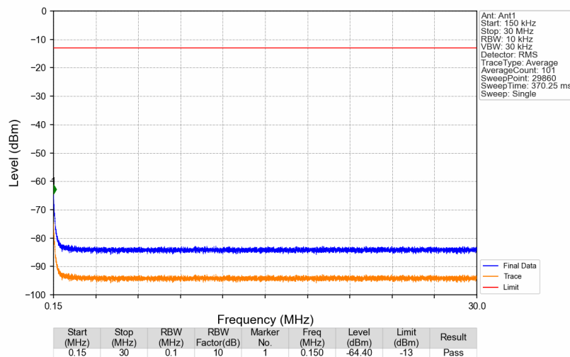
Band13_746.1MHz_GMSK_SISO_Ant1_NTNV
