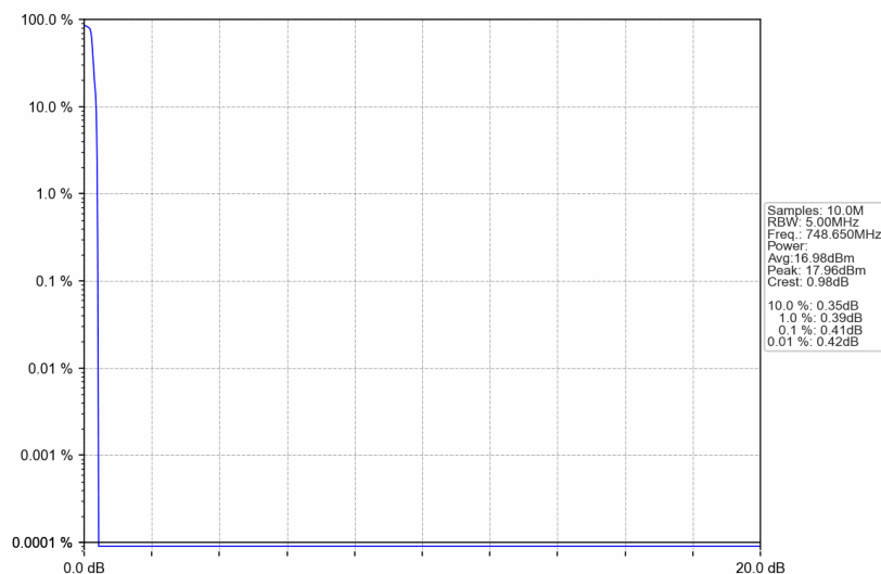
Band13_748.65MHz_GMSK_SISO_Ant1_NTNV_AGC
